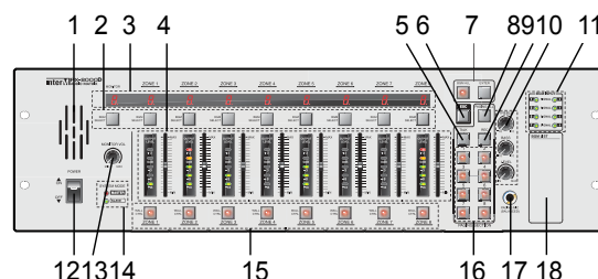
Передняя панель
