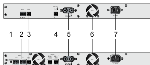
Задняя панель
