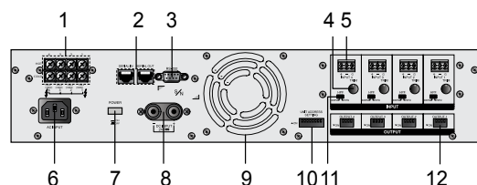
Задняя панель
