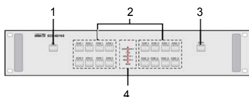
Передняя панель
