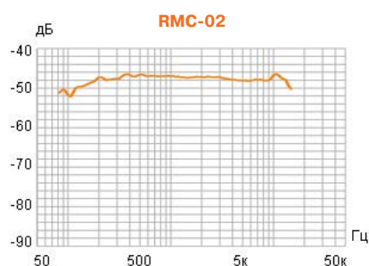
Амплитудно-частотная характеристика
