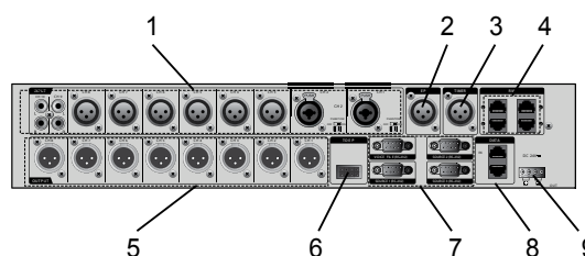
Задняя панель
